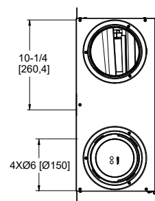
VOLET MOTORISÉ
