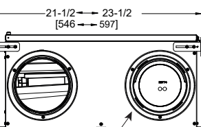
VOLET MOTORISÉ
