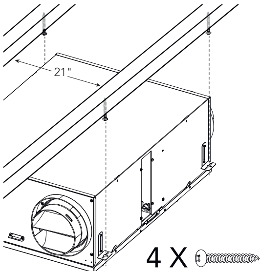
Instalación en techo
