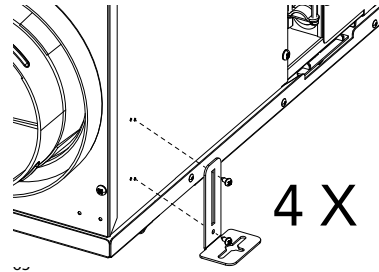
Instalación en la pared
