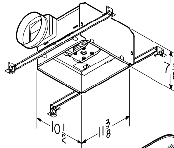
Models QTXEN080FLT, QTXEN110FLT
