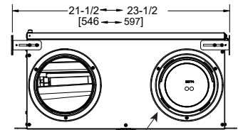
VOLET MOTORISÉ
