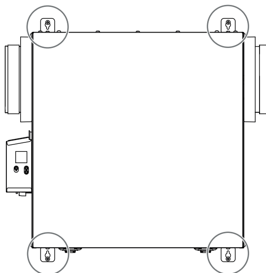
INSTALACIÓN CON 4 SOPORTES
